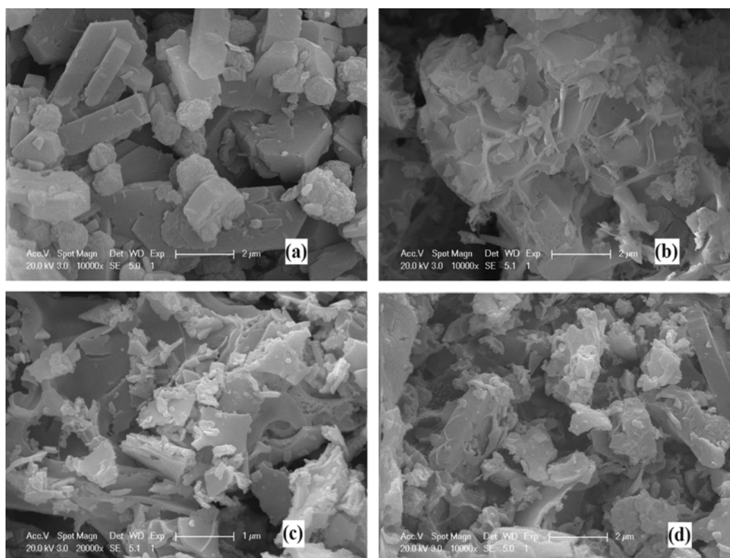
Fig. 1. SEM images: (a) ZSM-5 (b) fresh 5Ce5La/ZSM-5 (c) used 5Ce5La/ZSM-5 (d) regenerated 5Ce5La/ZSM-5.
